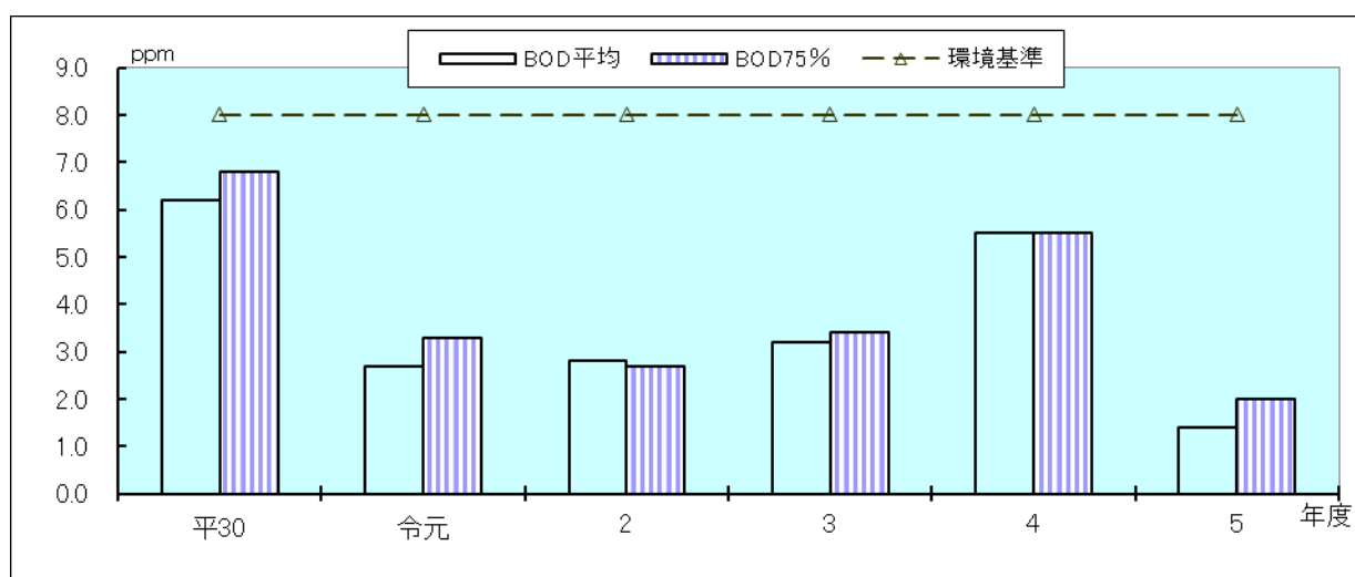
図3-2-6 山田川下流のBOD経年変化
