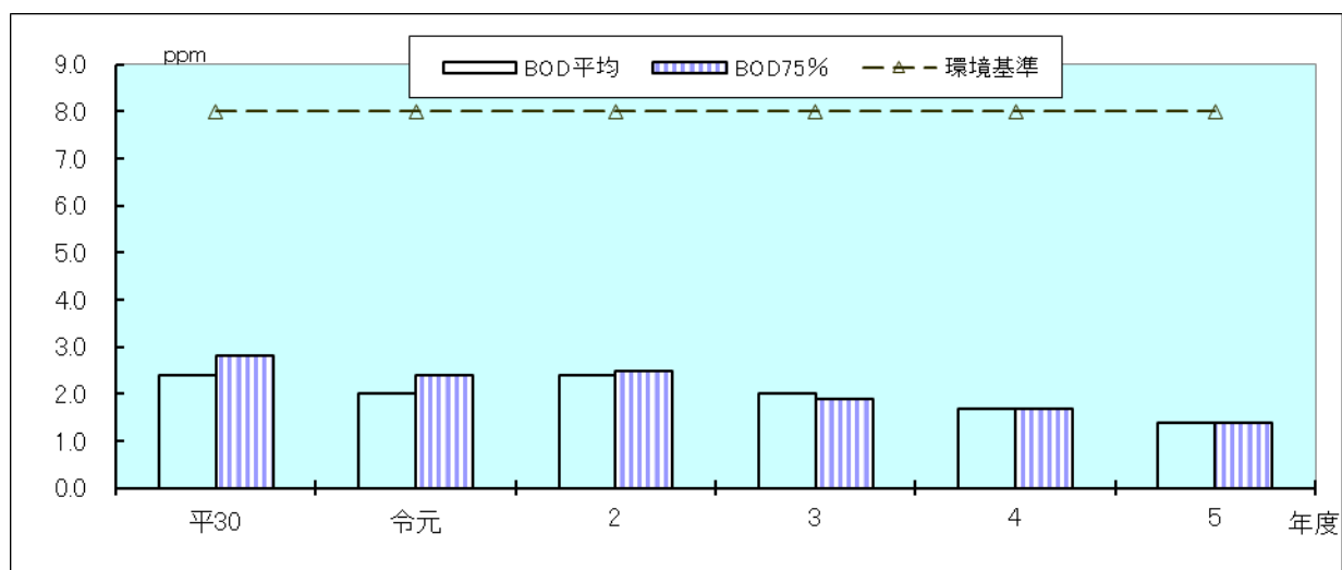
図3-2-5 日方川下流のBOD経年変化
