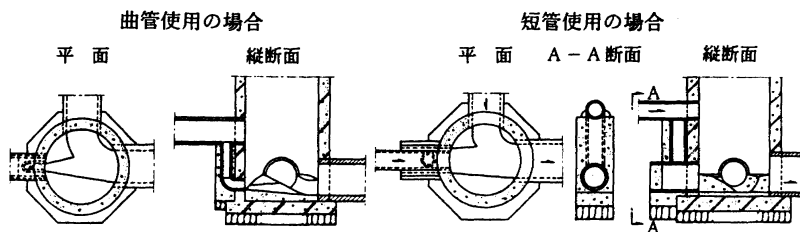
(1) 外副管設置構造図
