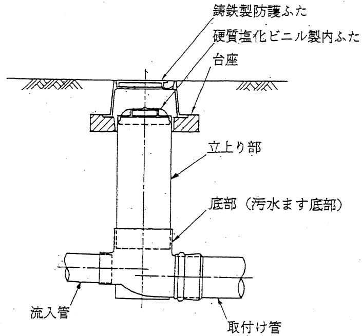
(参考図2) 雨水樹及び汚水樹の防護蓋の設置例
