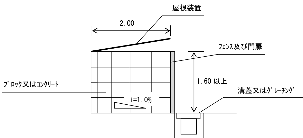
断面図
