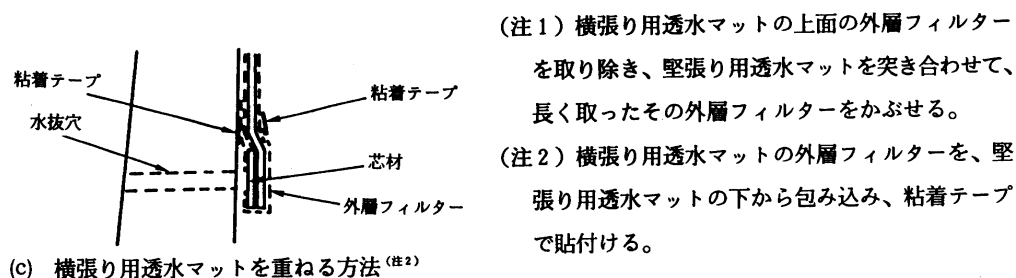
解説図 3-7 接続部の処理方法の例
