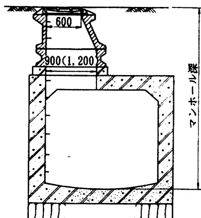
横断面
