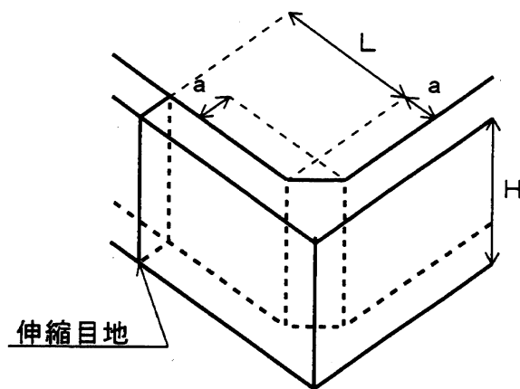
錬積み造擁壁の場合
