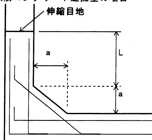
鉄筋コンクリート造擁壁の場合
