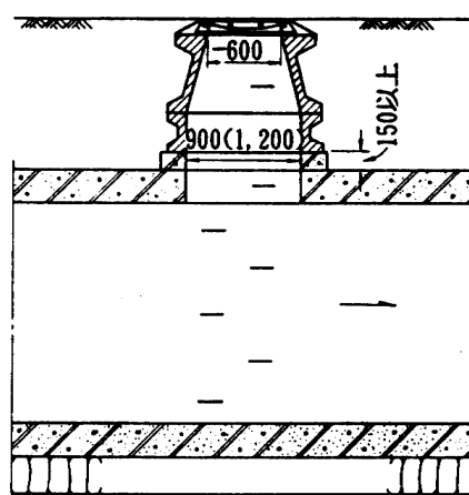
縦断面
