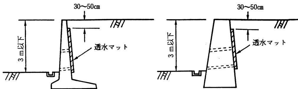
(a) 擁壁の高さが3 m以下の場合
