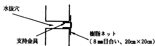
(a) 樹脂ネットを利用する方法
