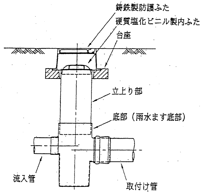
硬質塩化ビニル製雨水ます
