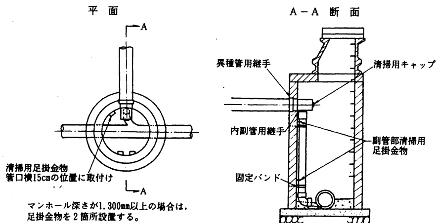
(2) 内副管設置構造図
