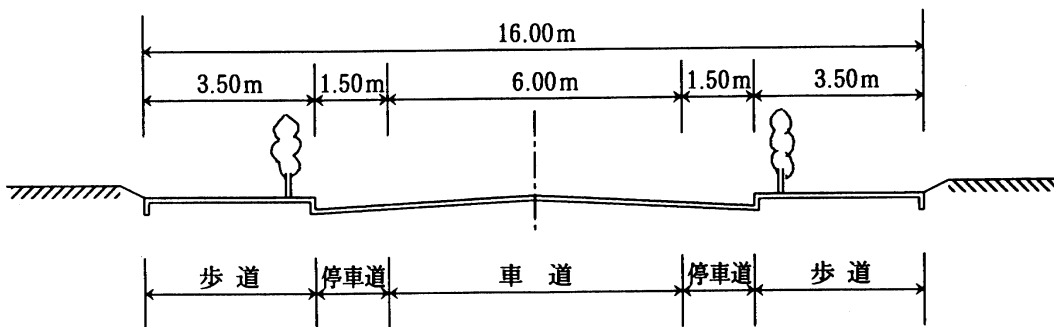
(e) 幅員 16.00m
