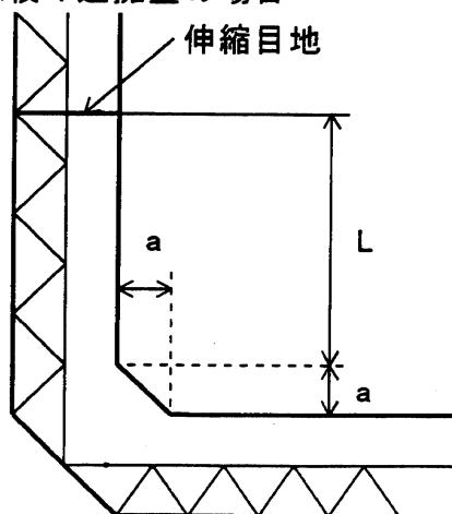
錬積み造擁壁の場合
