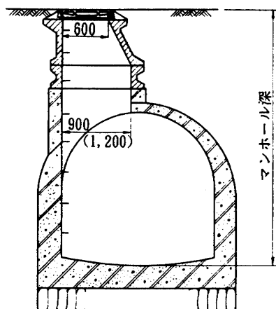
横断面
