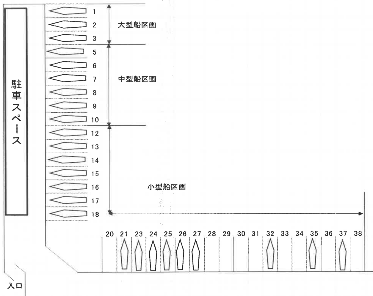
【冷水地区係留施設平面図】
