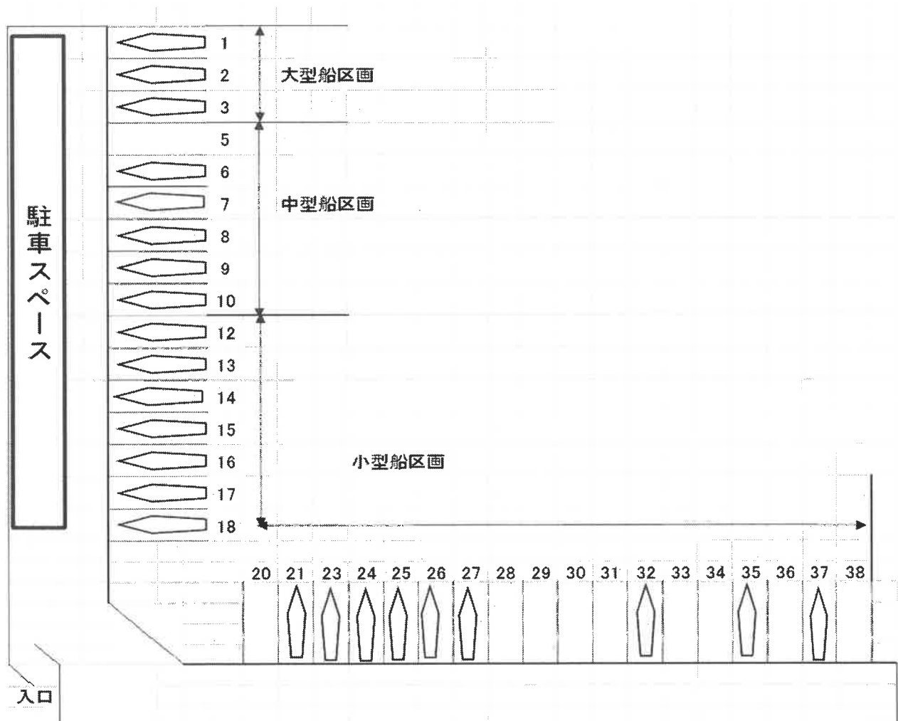
【冷水地区係留施設平面図】
