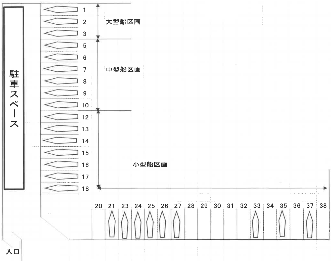
【冷水地区係留施設平面図】
