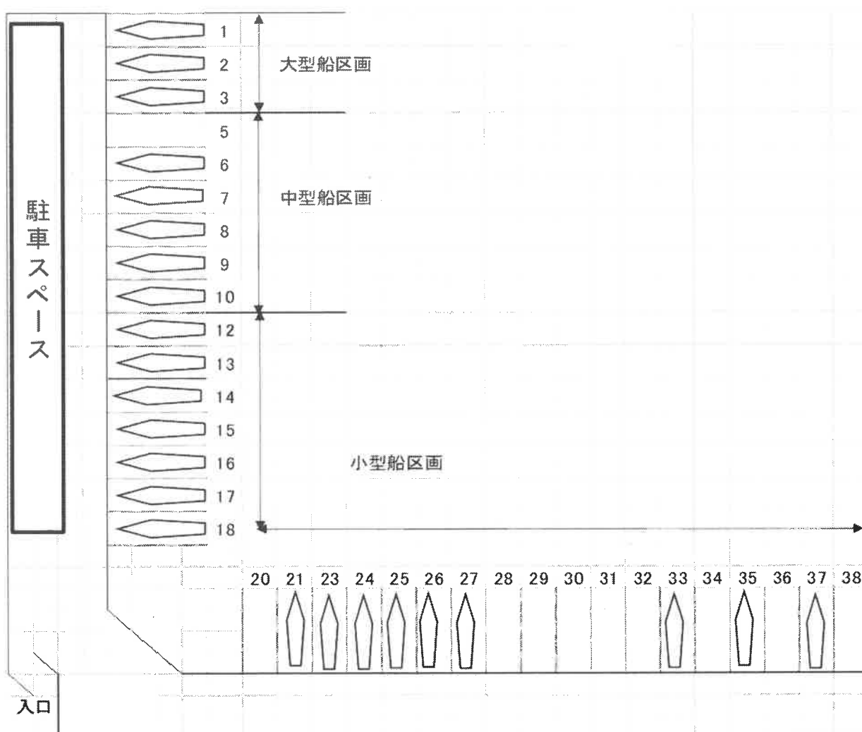
【冷水地区係留施設平面図】
