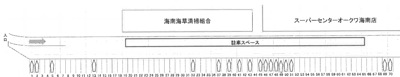
【築地地区係留施設平面図】
