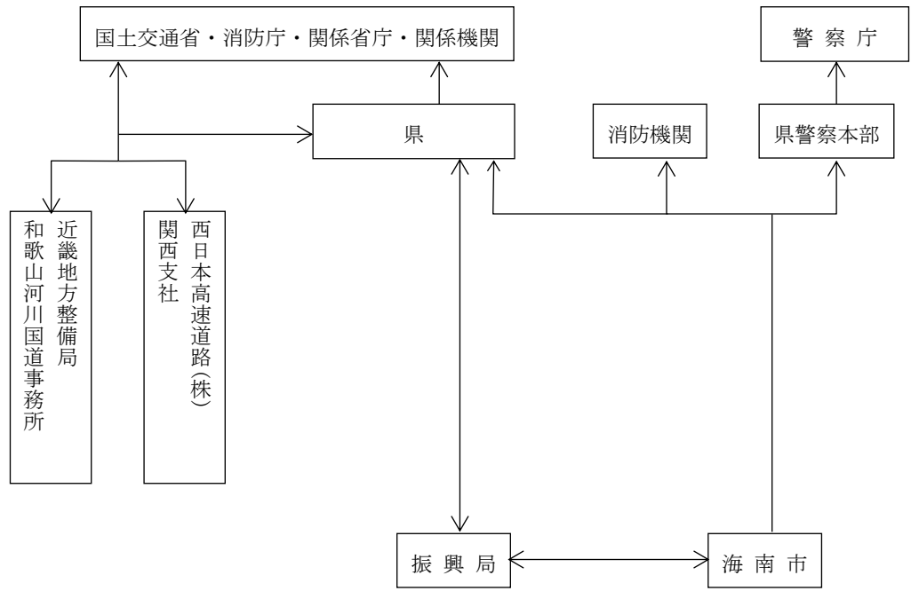
資料- 135 道路災害発生時の伝達系統
