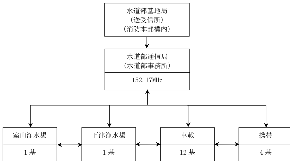
資料- 80 水道無線構成図
